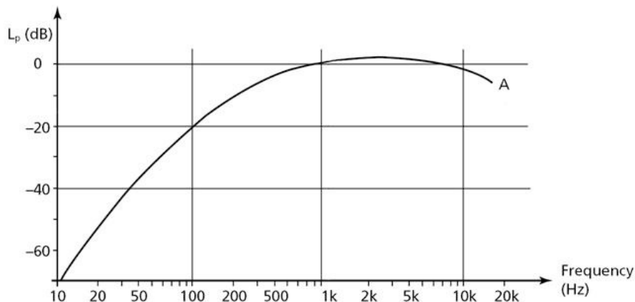
Figure 5 : Courbe de pondération fréquentielle A
